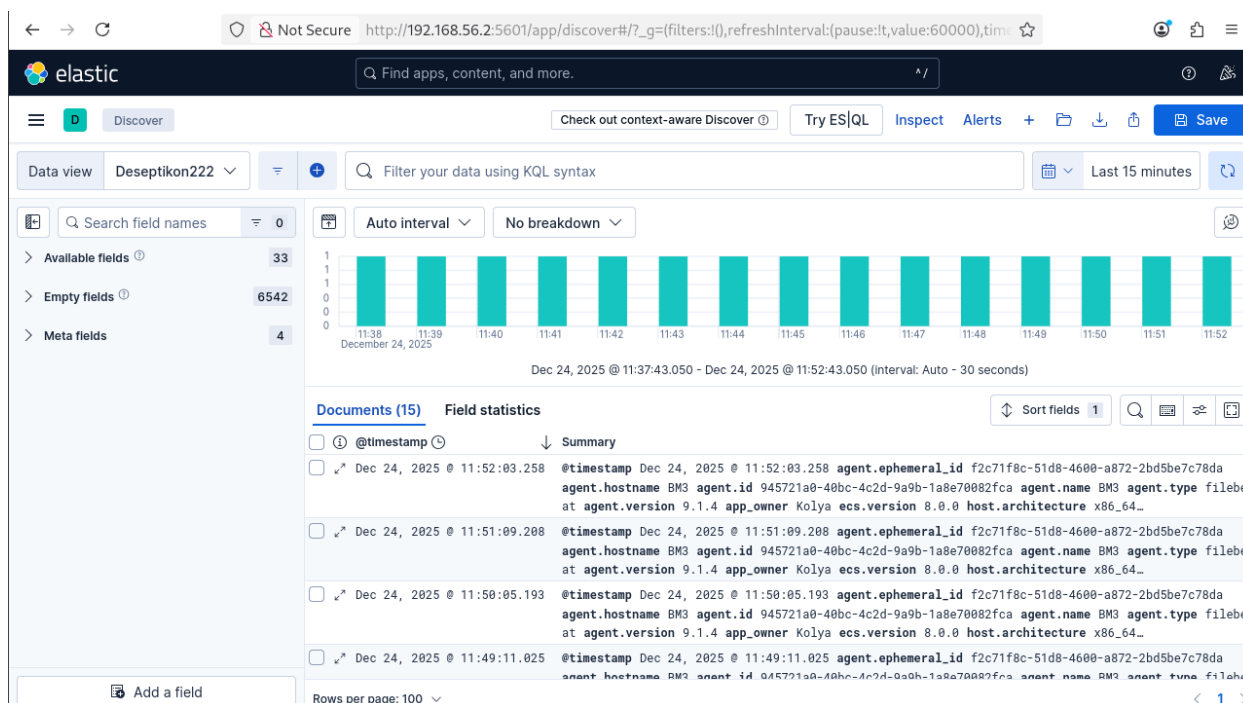
Рисунок 5 – Логи
