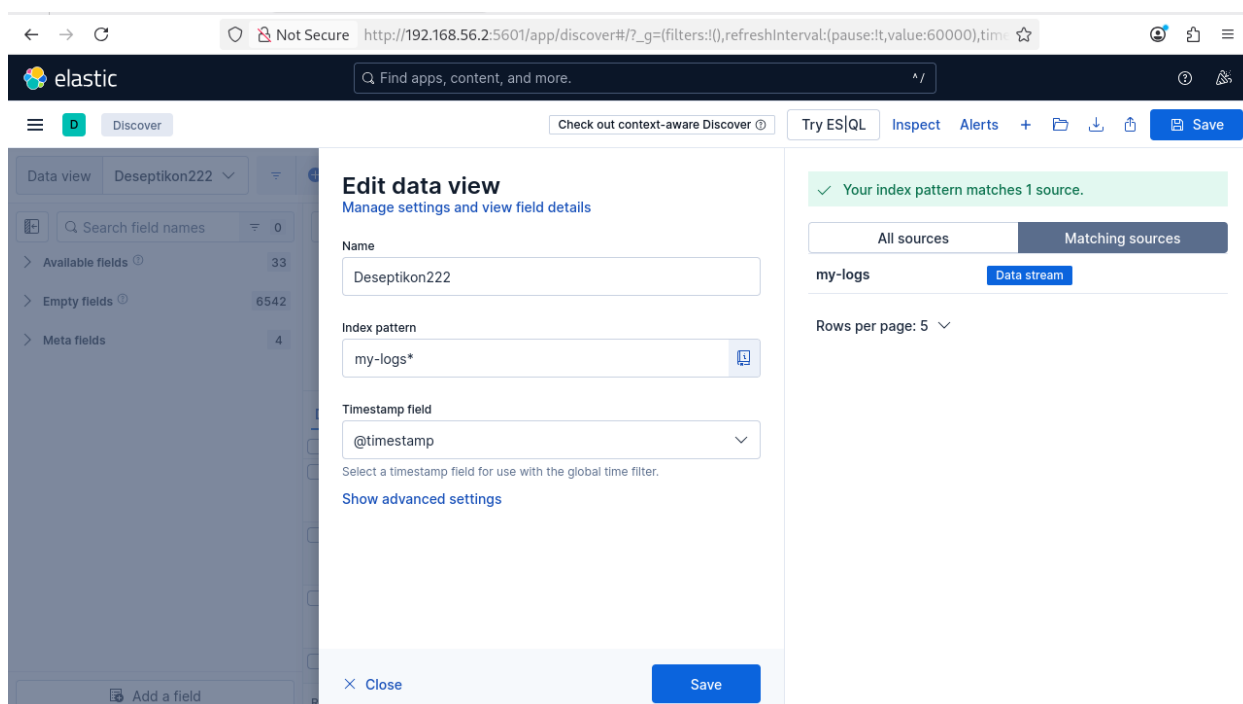
Рисунок 4 – Data view
